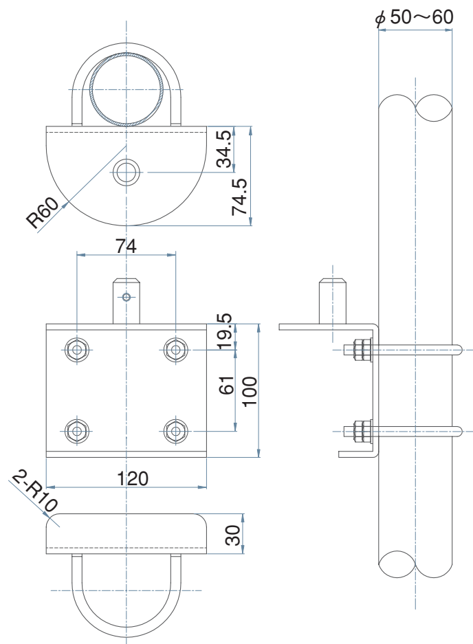
▲PS4-903 (適用パイプ径50~60mm)
